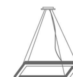
MD 103508-24B Длина 47см. Ширина 47см. Максимальная высота 120см. Количество источников света 24. Мощность 1W. Тип: светодиоды.
