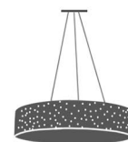
MD 9113-6E Диаметр 60см Максимальная высота 120см Количество ламп 6 Мощность max 13W Тип: лампа энергосберегающая Цоколь E14
